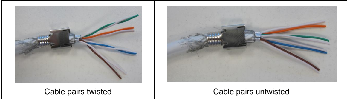
Figure 4. Untwist Cable Pairs
